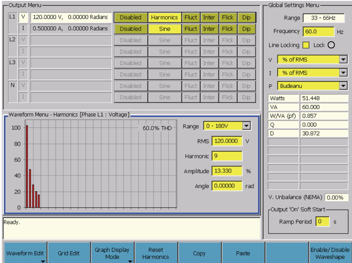
Рис. 4-13. Режим гармоник с частотным спектром сигнала
