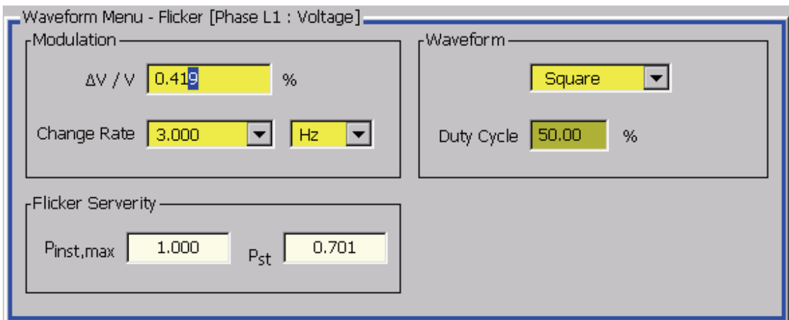
Рис. 4-30. Меню фликера (частота)
